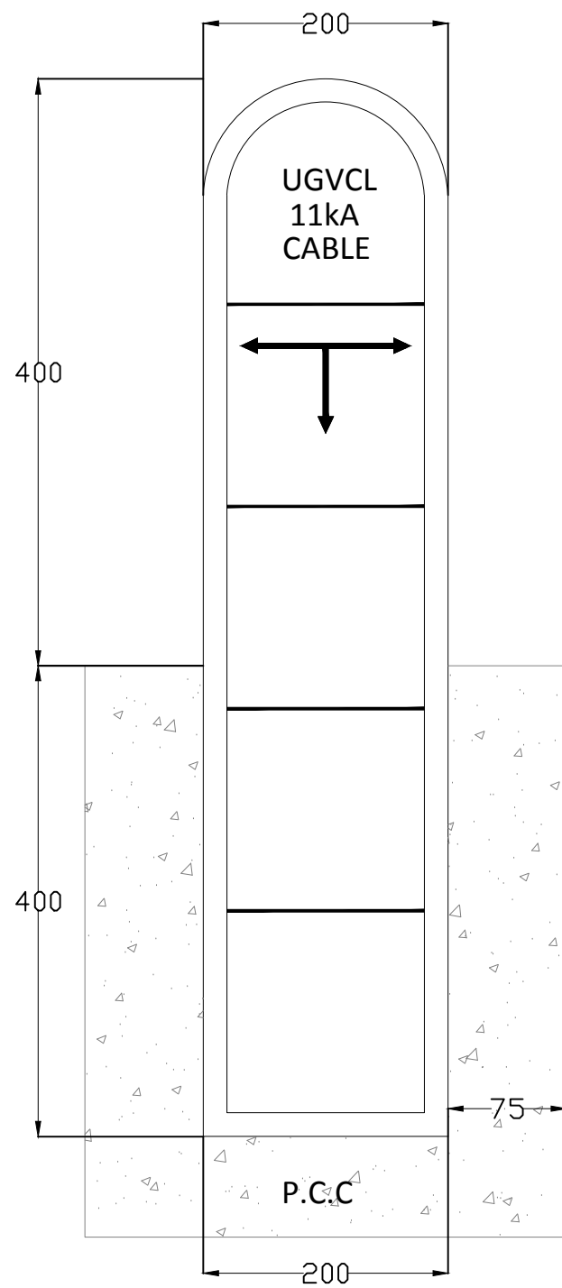
ELEVATION
